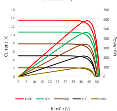
Curvas de corrente-tensão e potência-tensão (580W)
